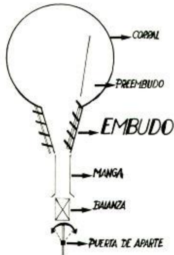
Figura 30: Pre-embudo y embudo
