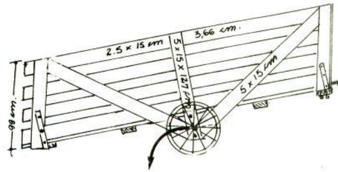
Figura 33: Cargador móvil con sistema para ajustar altura de embarque
